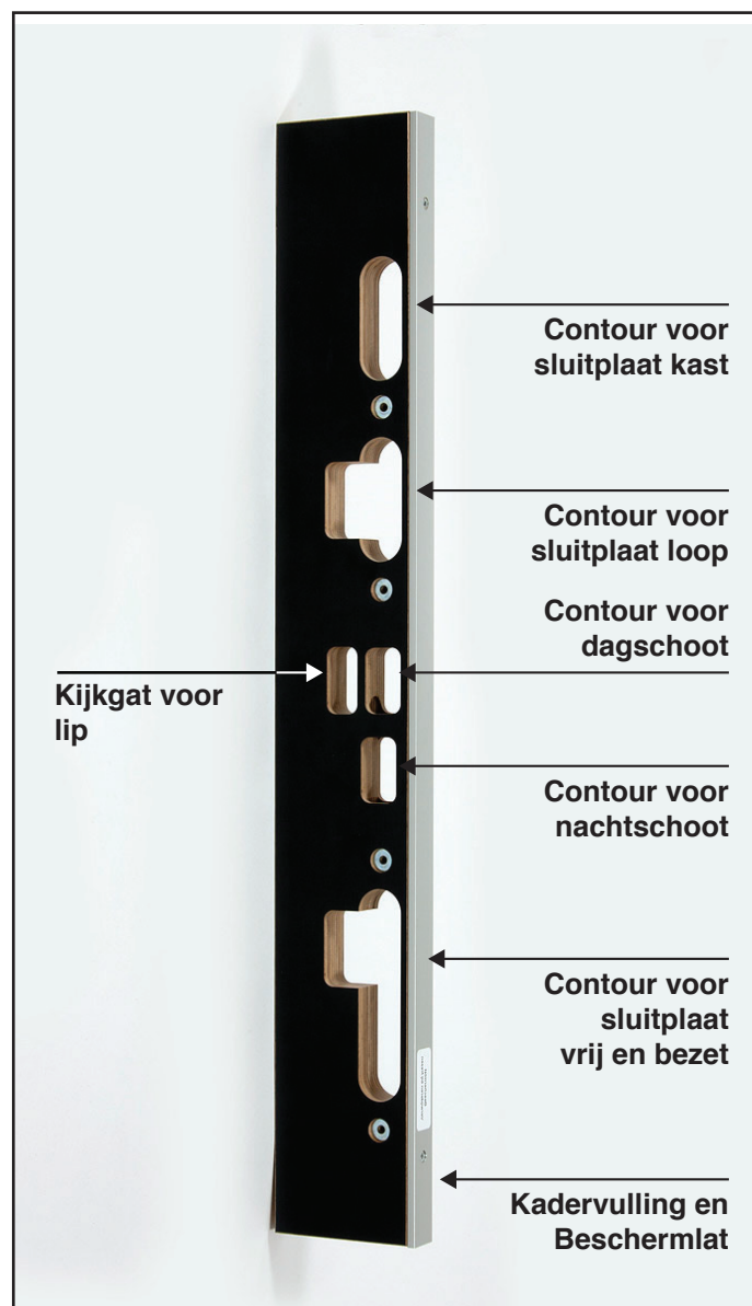
afb. 1 - Sluitplaat freesmal
